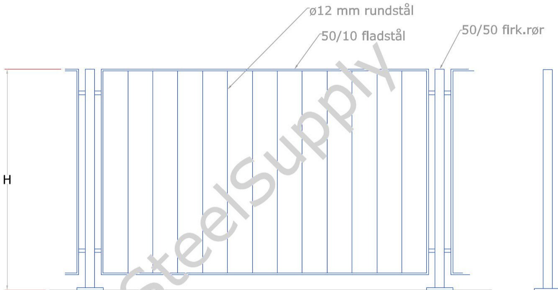
Rækværk type 5
